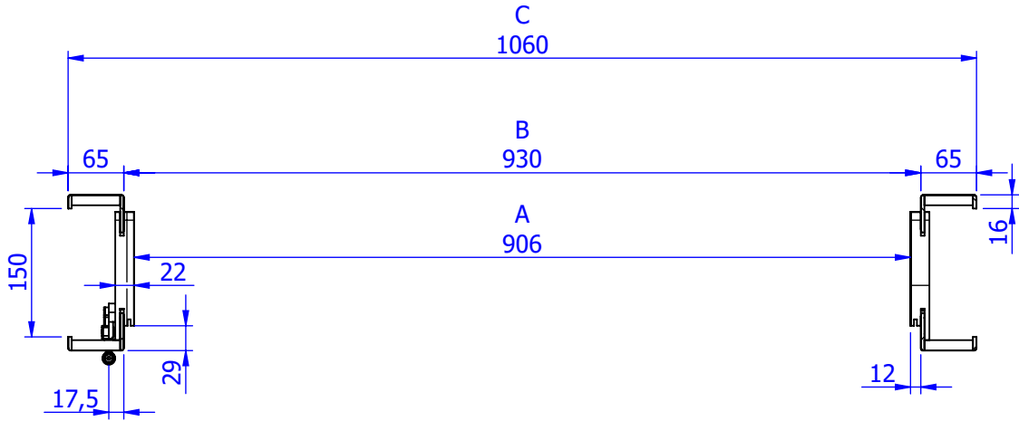
ŘEZ C-C MĚŘÍTKO 1 : 8
