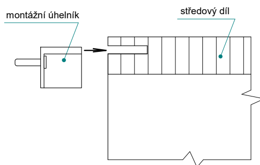
Řez zárubní
