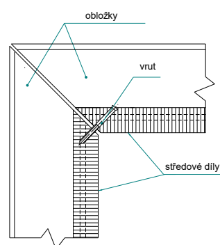
Řez zárubni
