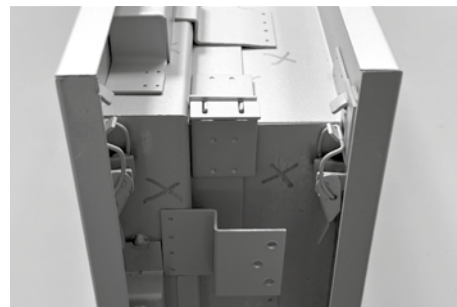
Kompletná zárubňa.
